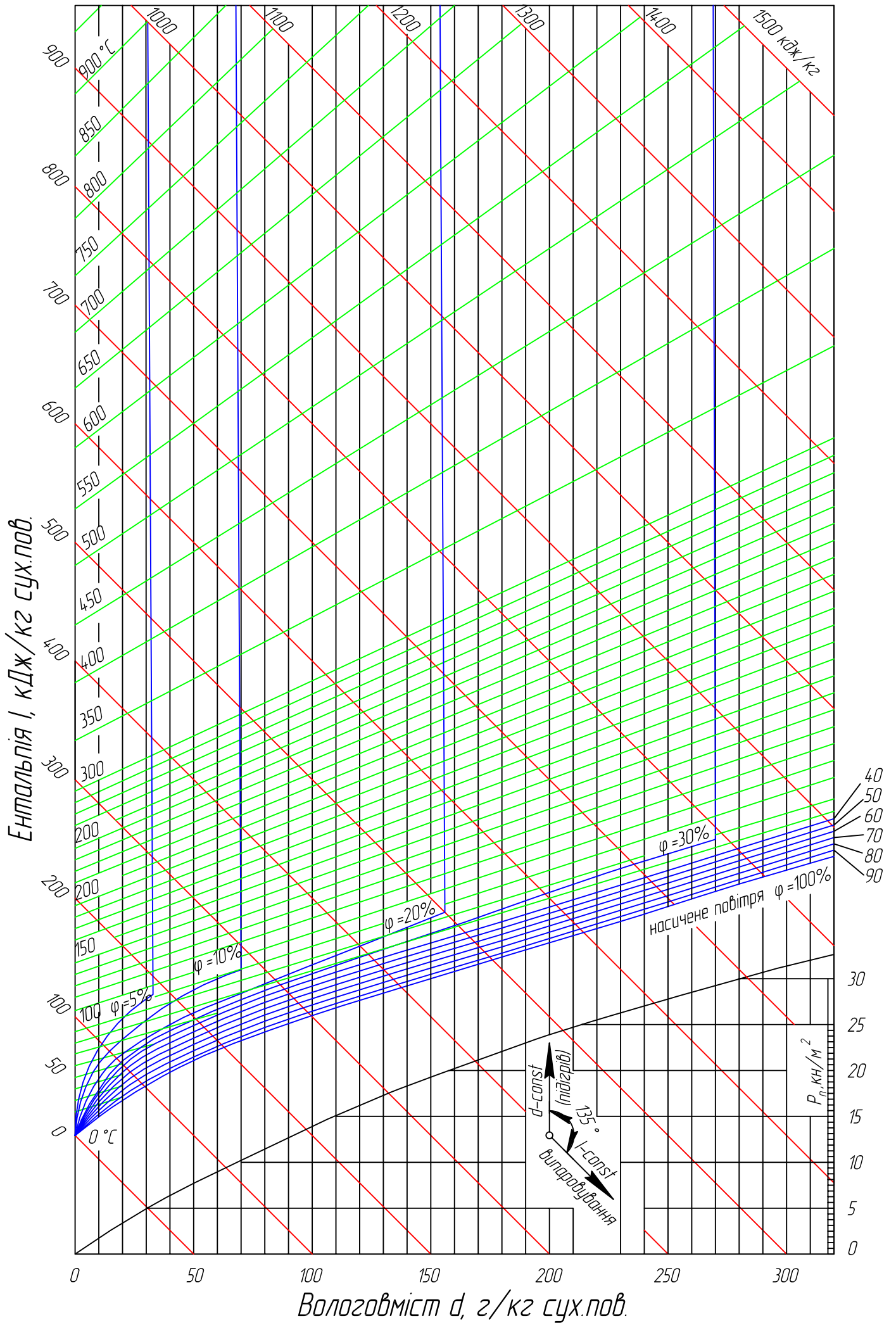
l-d- діаграма вологого повітря (до 800 °C) при барометричному тиску 99,4 кПа
